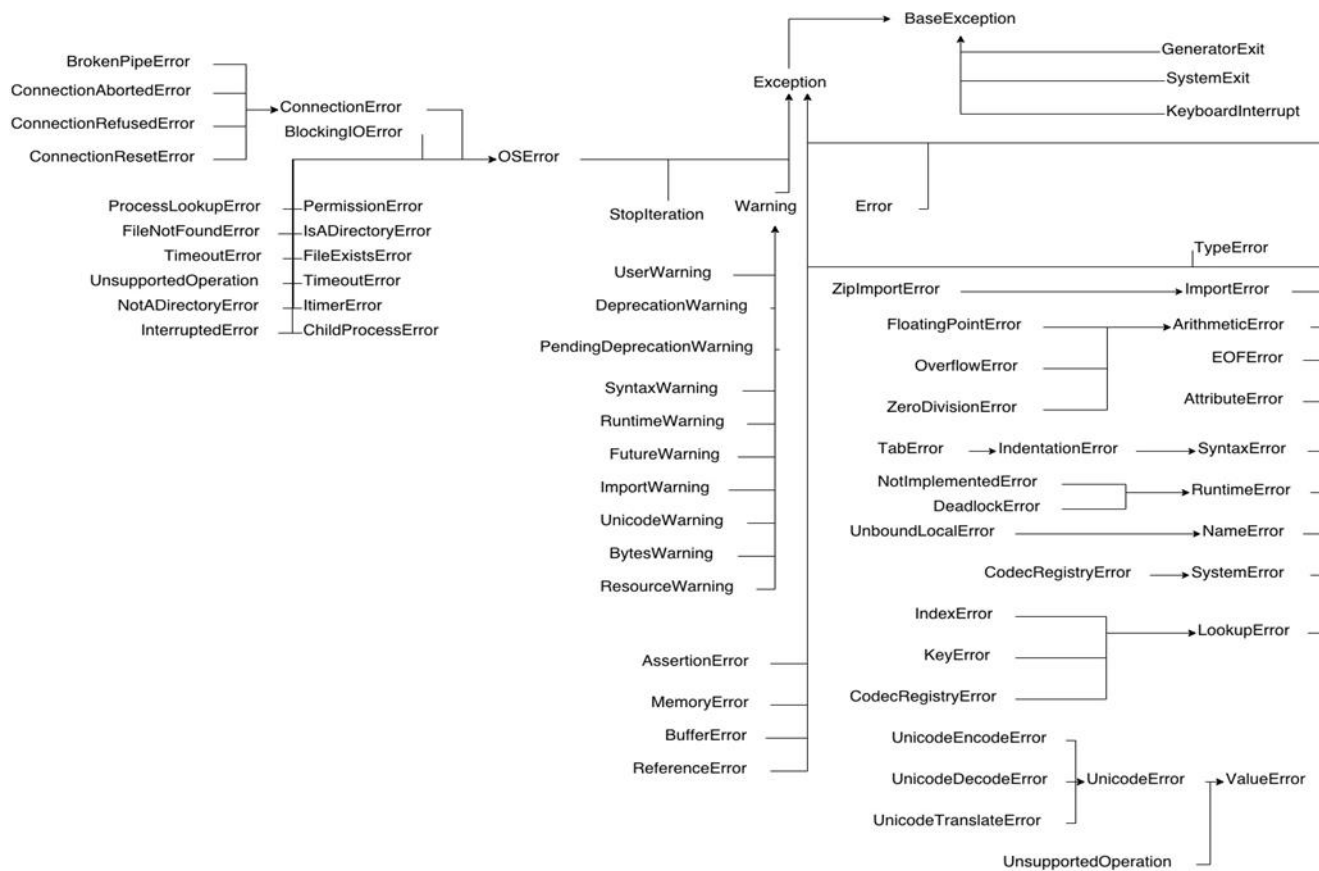
Сурет 19 – Python3-тің сатылық(иерархиялық) ерекшеліктері
